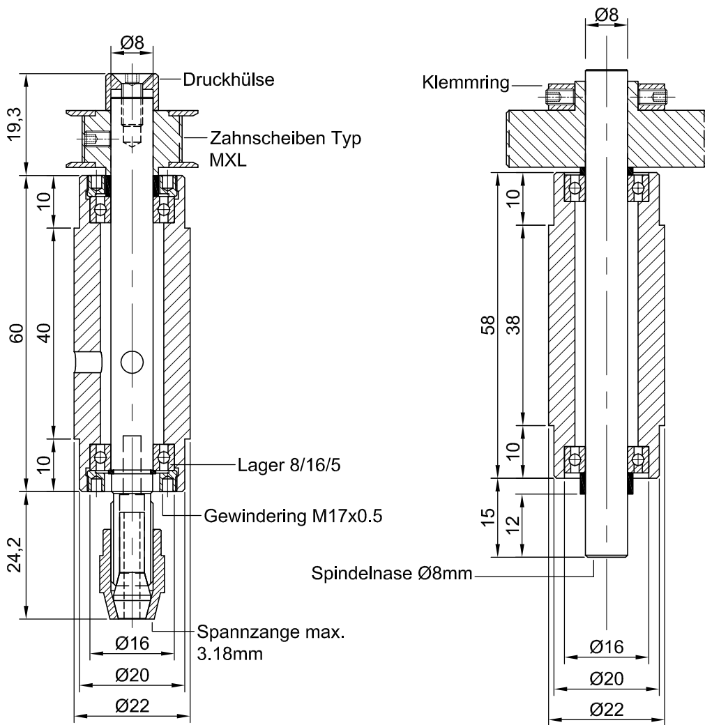
Schnell-Läufer Spindel
